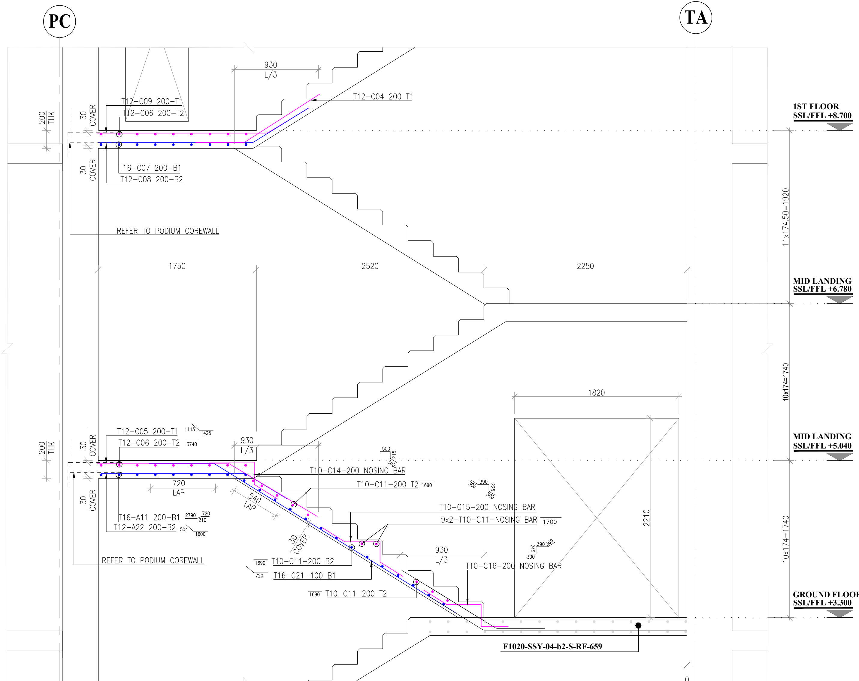
SECTION 1A-1A SCALE: 1:25
